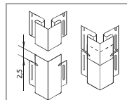
Рис. 3: Установка наружных и внутренних углов
